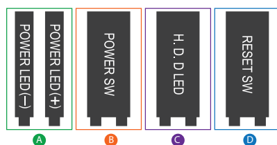
前面板导线
